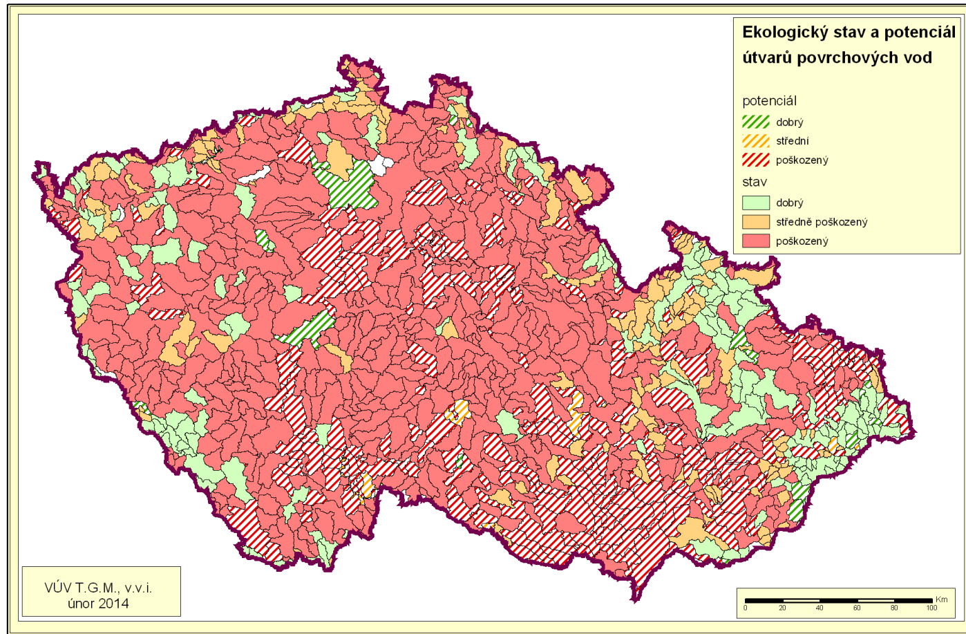
Obrázek 1: Ekologický stav a potenciál útvarů povrchových vod ČR
